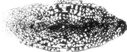
Beedeina megista Wahlman 2013
